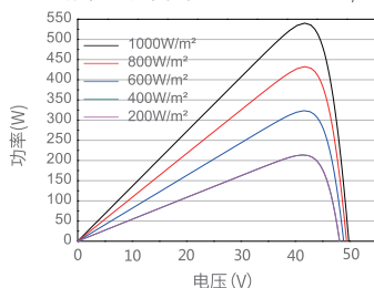
功率-电压曲线 JAM72S30-540/MR
